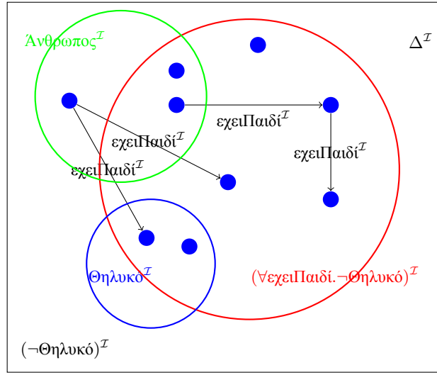
Σχήμα 1. Γραφική αναπαράσταση της ερμηνείας της έννοιας \top \sqcap \forall R.C \sqcap \neg \text{Θηλυκό}
